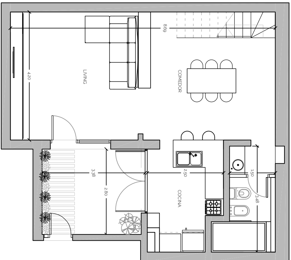
PLANTA BAJA 59 m 2 CUBIERTOS 9 m 2 PATIO
