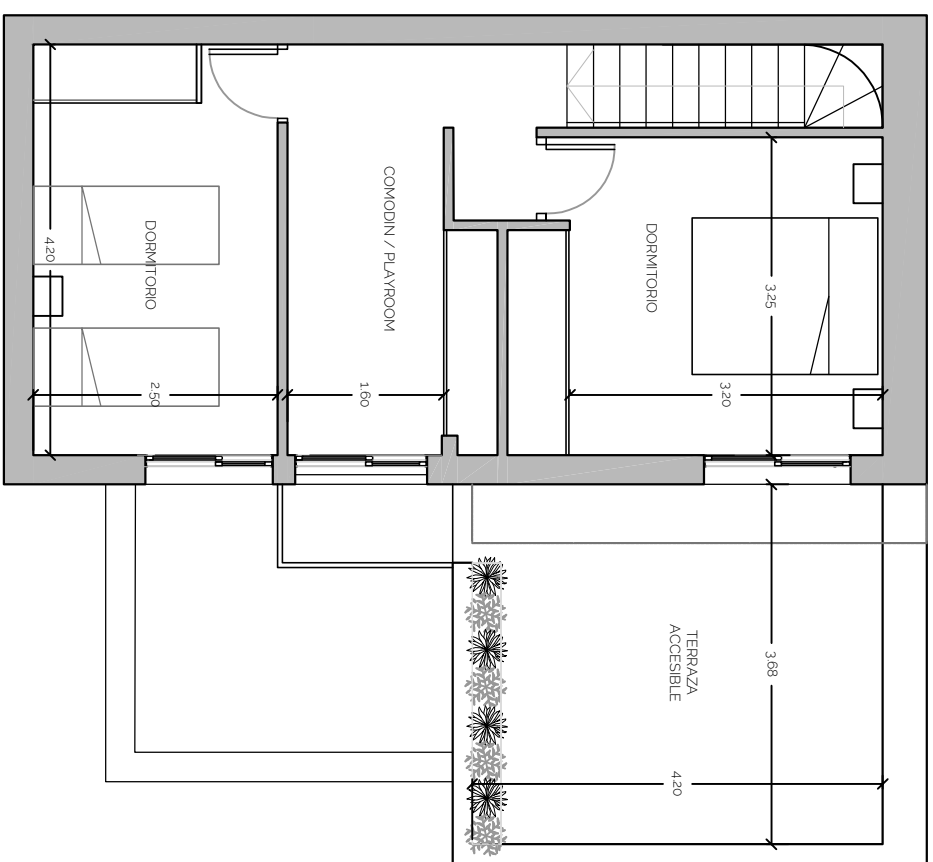
PLANTA ALTA 37 m 2 CUBIERTOS 15 m 2 BALCON/TERRAZA
