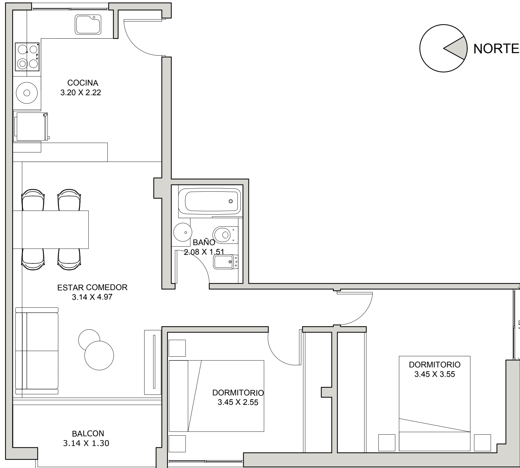
PLANTA esc 1:100
